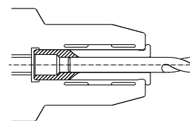
Desenho HSK-A/WD-CB
