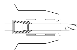
図面 HSK-A/WD-CB
