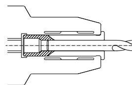
Zeichnung HSK-A/WD-CB
