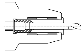
Dibujo 1 HSK-A/WD-CB
