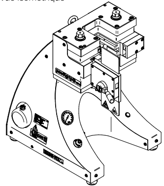
Vue isométrique
