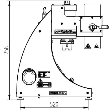
Vue du côté gauche
