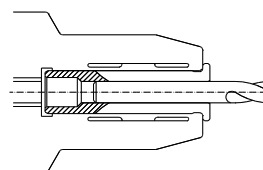
Dibujo 1 HSK-A/WD-CB
