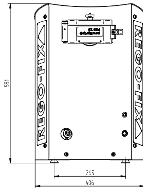
Ansicht Frontseite
