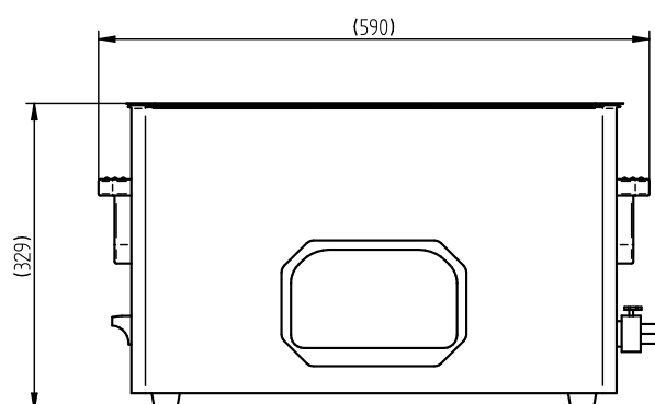
UCD 22 - 超音波洗浄機 22 リットル
