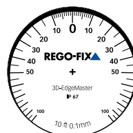
Cadran et tige disponibles en version métrique et version en pouce
