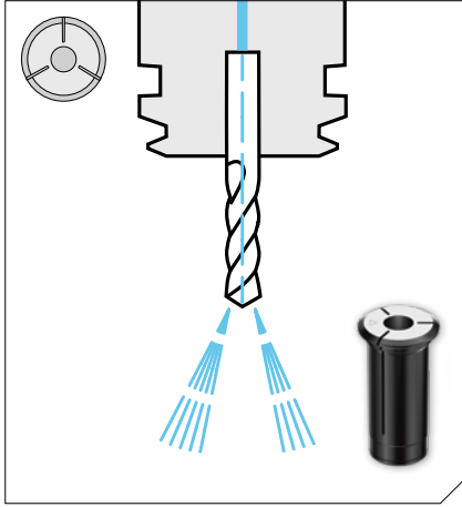
標準コレット:センタースルー
