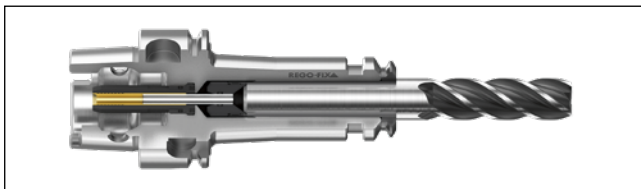
Kühlschmierstoffrohr KSR
