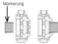
Kühlscheibe KS
